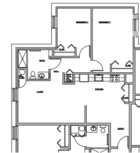
TYPE A - 2 BEDROOM UNIT SCALE: 1/8" = 1'-0"
