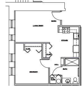
TYPE E - 1 BEDROOM UNIT SCALE: 1/8" = 1'-0"
